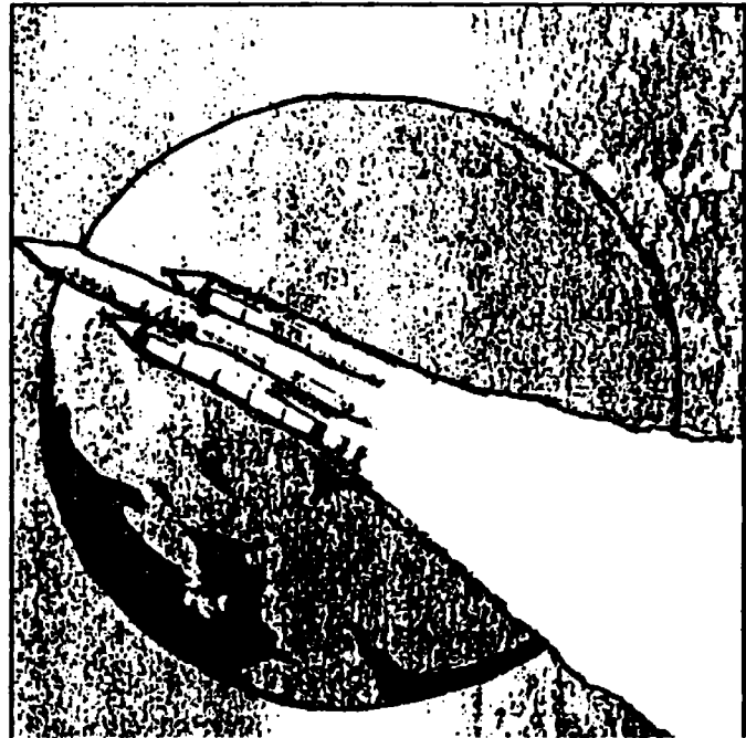
صورة الأرض من الفضاء الخارجي تبين أن الأرض كروية الشكل
